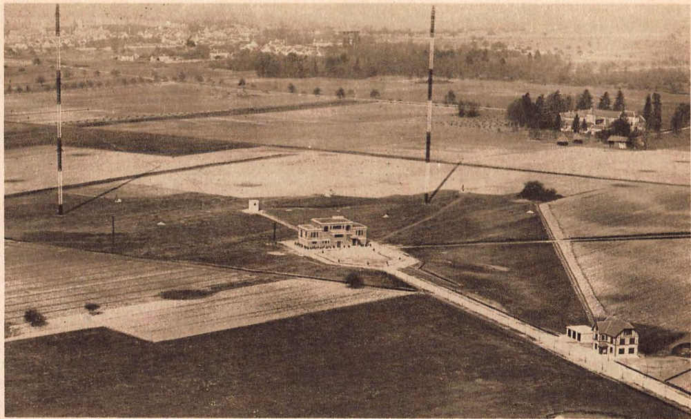
POSTE PARISIEN. — Vue aérienne de la station des Molières (S.-et-O.) Longueur d'onde : 312 mètres 80. — Puissance : 60 kilowatts. — Fréquence : 959 kilocycles
